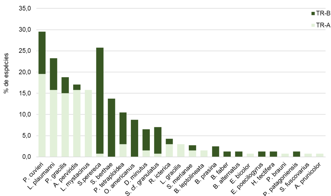
GRÁFICO 8 – PORCENTAGEM DAS ABUNDÂNCIAS DE ESPÉCIES DE ANUROS REGISTRADAS NA ÁREA TR-A E ÁREA TR-B DURANTE A DÉCIMA CAMPANHA.
