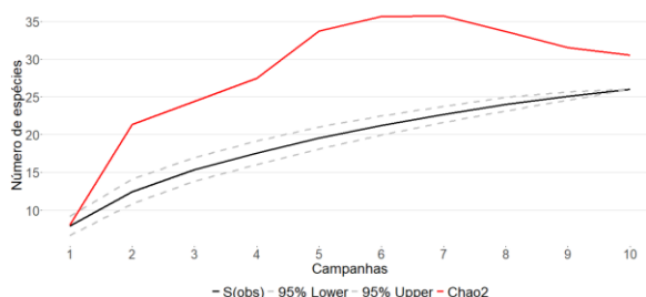
GRÁFICO 25 – CURVA DE RAREFAÇÃO PARA AS ESPÉCIES DE MAMÍFEROS REGISTRADAS POR TODOS OS MÉTODOS NO MÓDULO TR-A (ÁREA-CONTROLE) DURANTE AS DEZ CAMPANHAS NA PCH TRÊS CAPÕES NOVO, GUARAPUAVA/PR.
