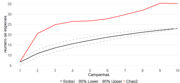
GRÁFICO 26 – CURVA DE RAREFAÇÃO PARA AS ESPÉCIES DE MAMÍFEROS REGISTRADAS POR TODOS OS MÉTODOS NO MÓDULO TR-B (ADA) DURANTE AS DEZ CAMPANHAS NA PCH TRÊS CAPÕES NOVO, GUARAPUAVA/PR.
