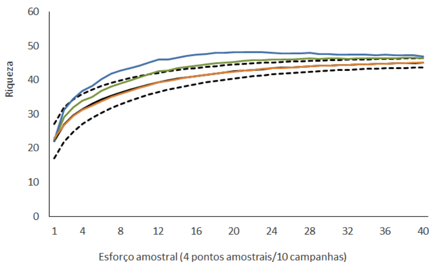
GRÁFICO 31 - CURVA DE RAREFAÇÃO DE ESPÉCIES (LINHA PRETA CONTÍNUA), INTERVALO DE CONFIANÇA (LINHAS TRACEJADAS) E RIQUEZA TOTAL PREVISTA PELOS ESTIMADORES BOOTSTRAP (LINHA VERDE), CHAO-1 (LINHA LARANJA) E JACKKNIFE-1 (LINHA AZUL) PARA O ESFORÇO AMOSTRAL DOS MACROINVERTEBRADOS AQUÁTICOS NAS CAMPANHAS DE MONITORAMENTO DA PCH TRÊS CAPÕES NOVO, NO RIO JORDÃO, GUARAPUAVA (PR).
