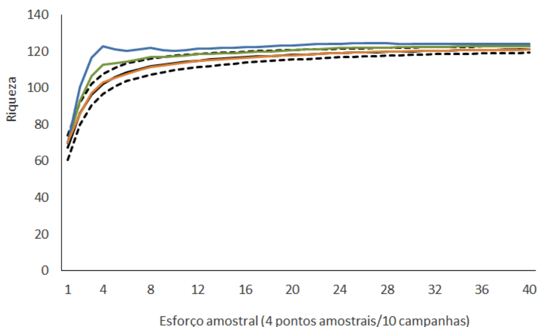
GRÁFICO 36 - CURVA DE RAREFAÇÃO DE ESPÉCIES (LINHA PRETA CONTÍNUA), INTERVALO DE CONFIANÇA (LINHAS TRACEJADAS) E RIQUEZA TOTAL PREVISTA PELOS ESTIMADORES BOOTSTRAP (LINHA VERDE), CHAO-1 (LINHA LARANJA) E JACKKNIFE-1 (LINHA AZUL) PARA O ESFORÇO AMOSTRAL DOS ORGANISMOS PLANCTÔNICOS NAS CAMPANHAS DE MONITORAMENTO DA PCH TRÊS CAPÕES NOVO, NO RIO JORDÃO, GUARAPUAVA (PR).
