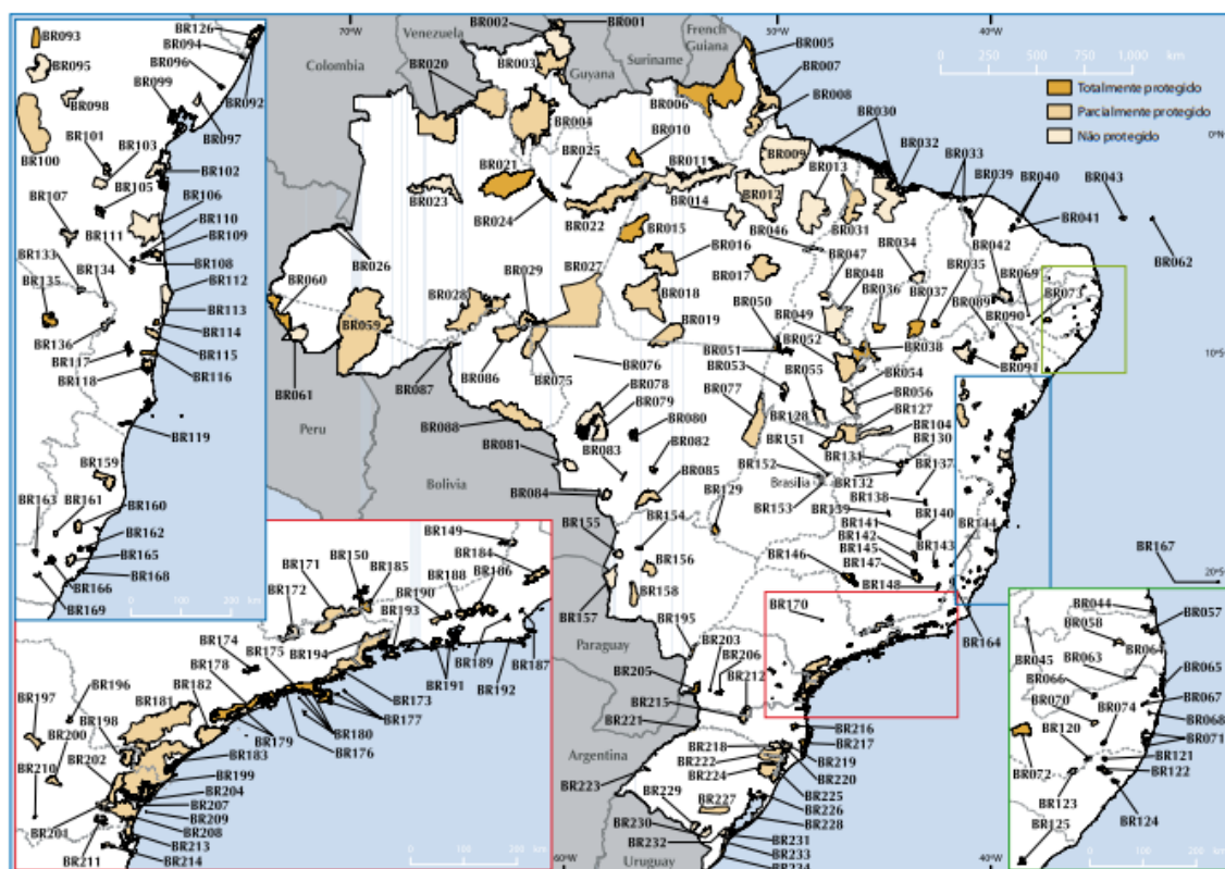
FIGURA 9 - MAPA DAS ÁREAS IMPORTANTES PARA A CONSERVAÇÃO DAS AVES NO BRASIL (IBAS).
