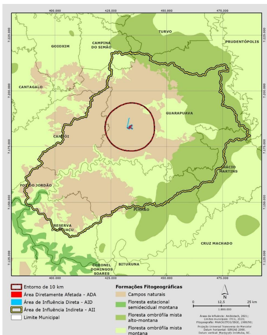
FIGURA 13 – MAPA COM AS FORMAÇÕES FITOGEográfICAS EXISTENTES NO ENTORNO DA REGIÃO ONDE SITUA-SE A PCH TRÊS CAPÕES NOVO.
