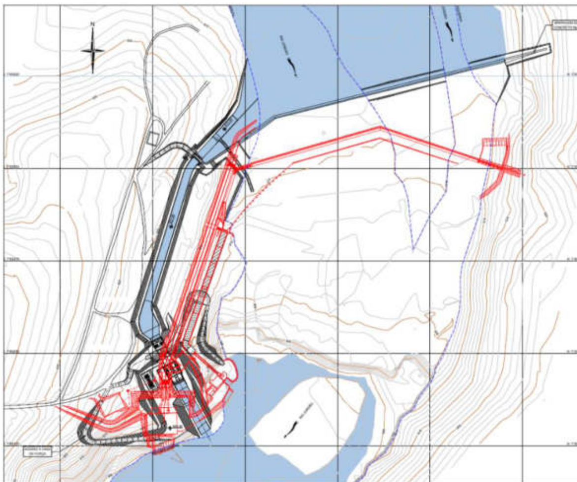
FIGURA 20 – COMPARATIVO PROJETO BÁSICO (2008 – COR VERMELHA) VERSUS PROJETO BÁSICO CONSOLIDADO (2021 – COR PRETA) DA PCH TRÊS CAPÕES NOVO.
