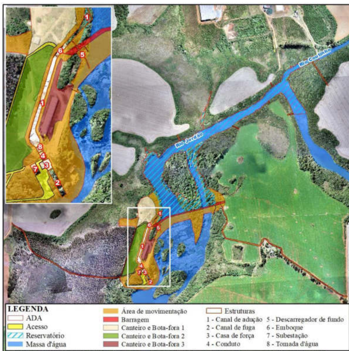
FIGURA 6 – ESTRUTURAS DA PCH TRÊS CAPÕES NOVO
